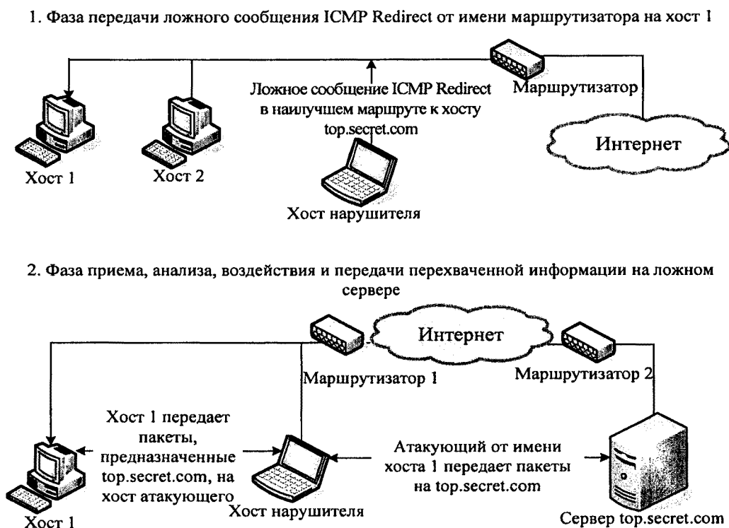
Рисунок 8. Схема реализации атаки "Навязывание ложного маршрута" (внутрисегментное) с использованием протокола ICMP с целью нарушения связи
