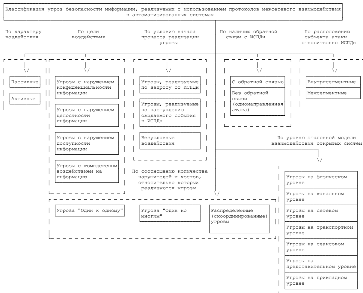
Рисунок 5. Классификационная схема угроз с использованием протоколов межсетевого взаимодействия
