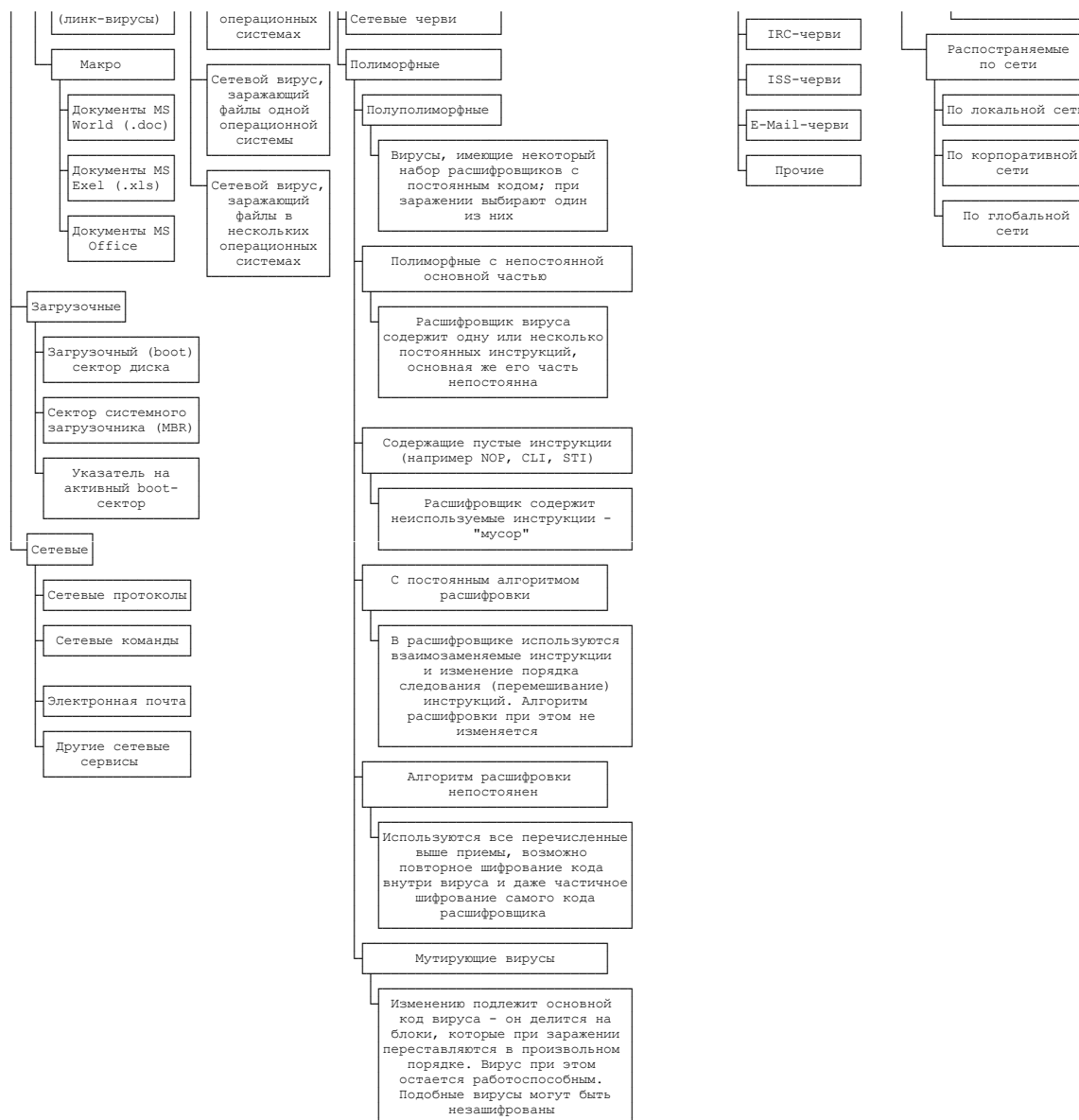
Рисунок 14. Классификация программных вирусов и сетевых червей
