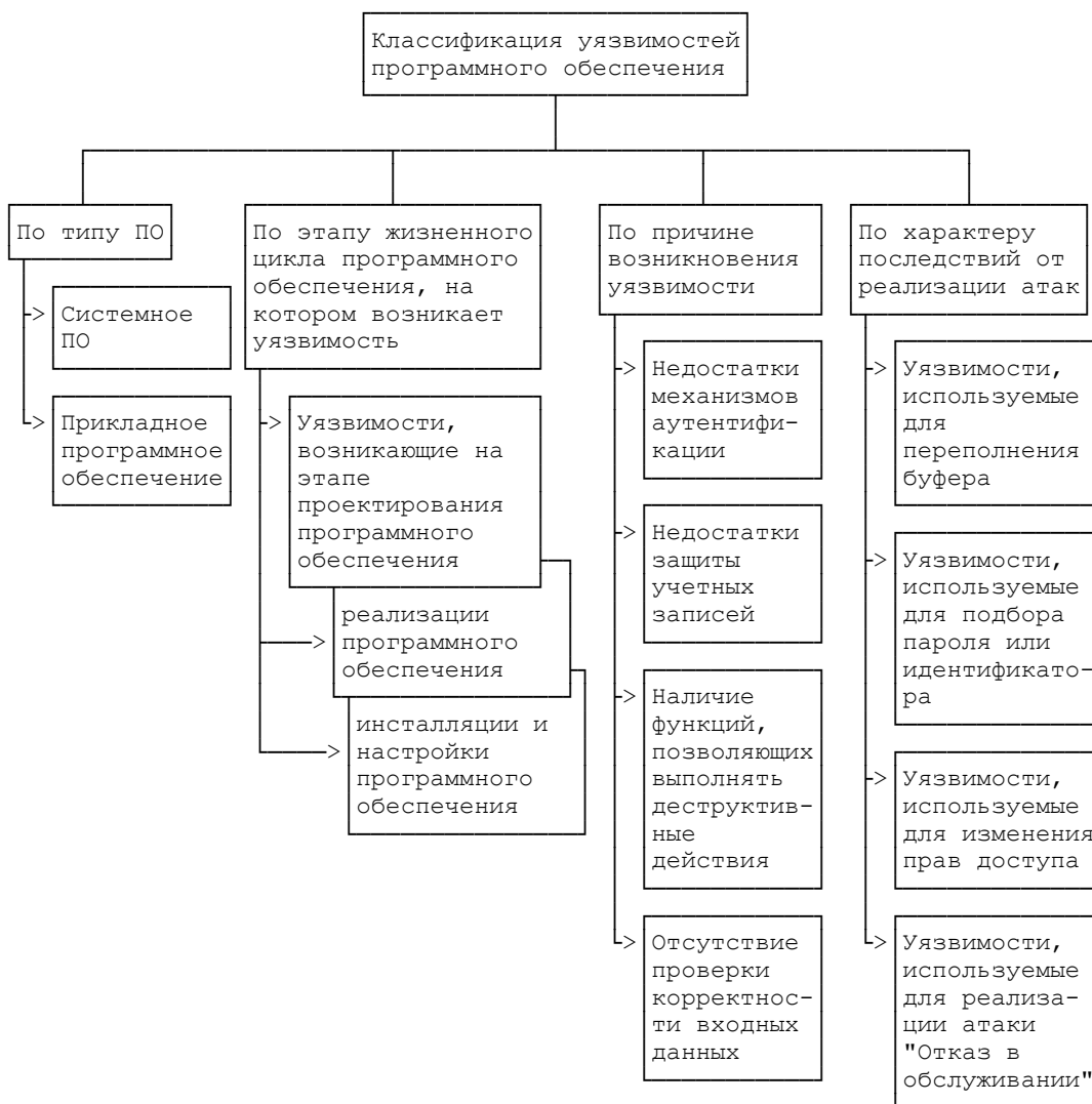
Рисунок 4. Классификация уязвимостей программного обеспечения
